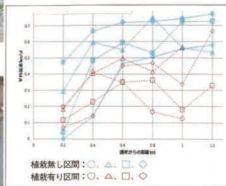
図5 護岸周辺の流速測定結果
