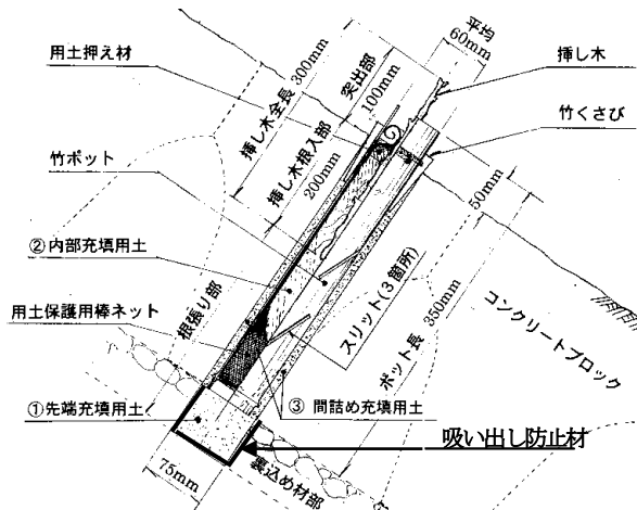
図-2 植栽孔への竹ポット構造体の挿入と固定
