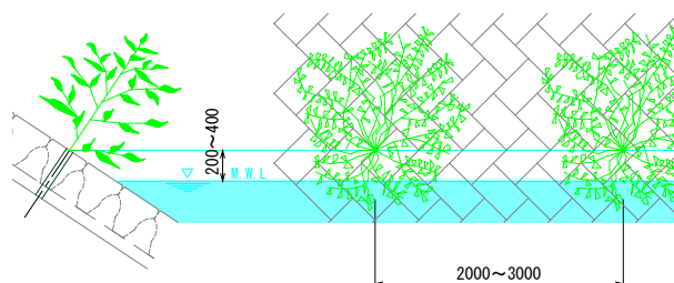
図-3 ネコヤナギの植栽高さと間隔の標準
